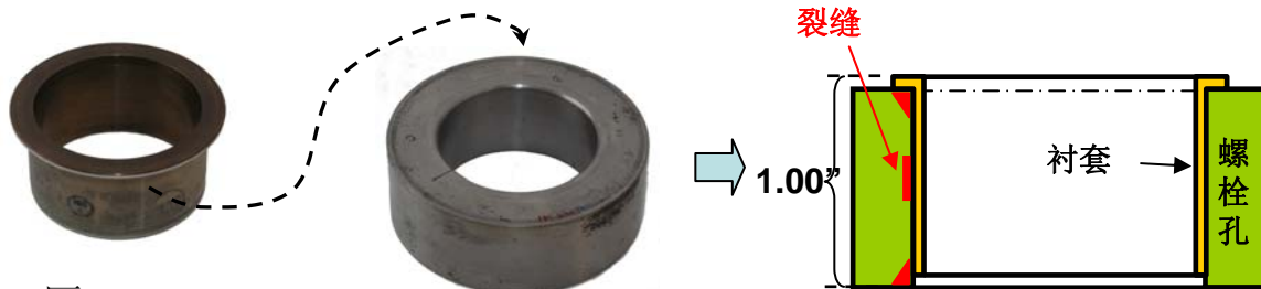
2mm厚 铝镍铜合金衬套
